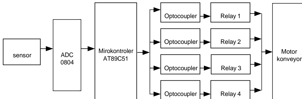
Gambar 3. Diagram blok rangkain kontrol
