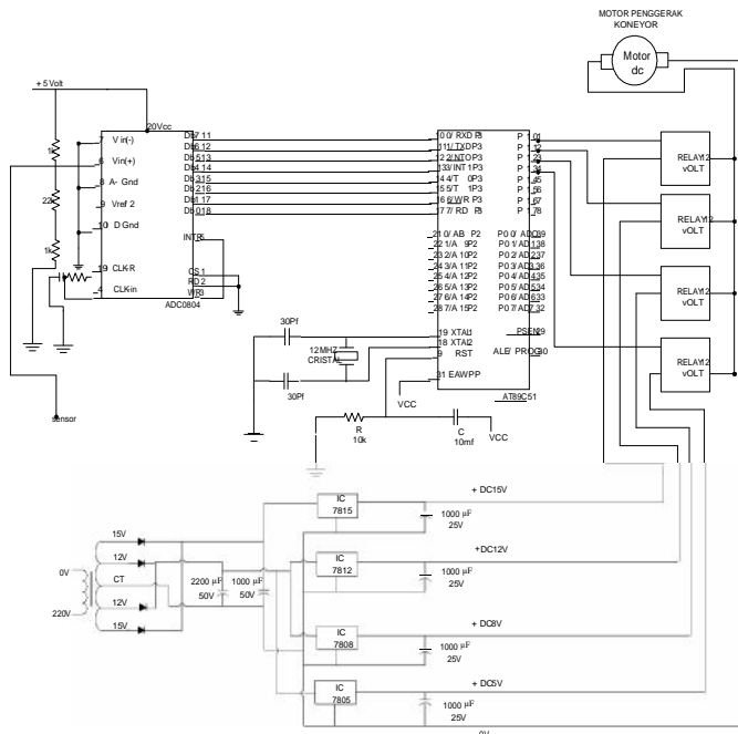
Gambar 7. Bentuk Rangkain Alat keseluruhan
