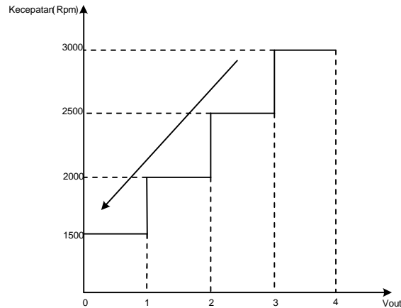
Gambar 9. Grafik perubahan kecepatan dengan tegangan yang dihasilkan
