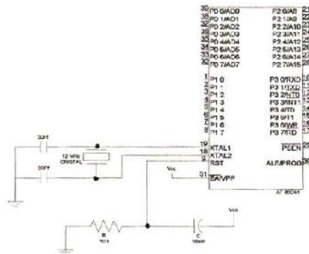
Gambar 5. Sistem minimum mikrokontroler AT89C51
