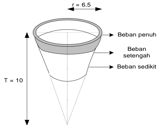
Gambar 10. Corong pada mesin giling
