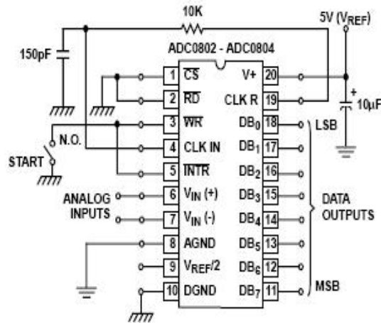
Gambar 4. Rangkain ADC0804
